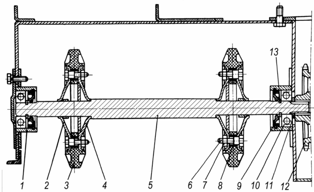
Рис. 6 – Ведущий вал гусениц
