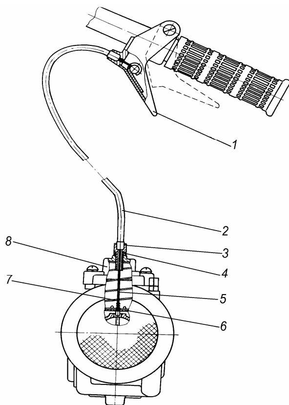
Рис. 13 – Привод управления дросселем карбюратора
