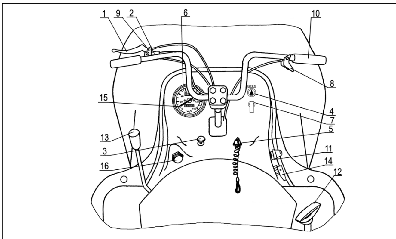
Рис. 11 – Органы управления (снегоходы БУРАН Л, ЛЕ, ЛД, ЛДЕ)
