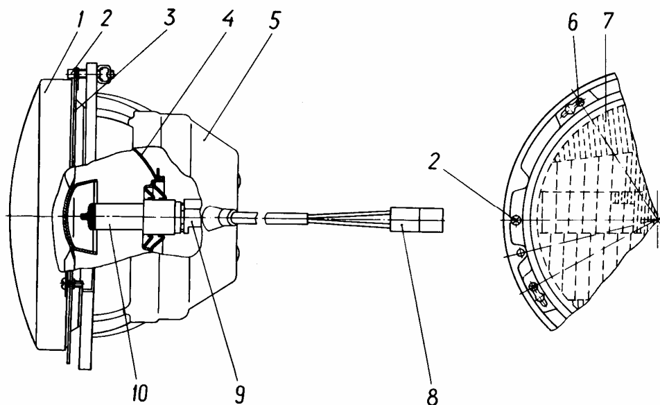
Рис. 16 – Фара
