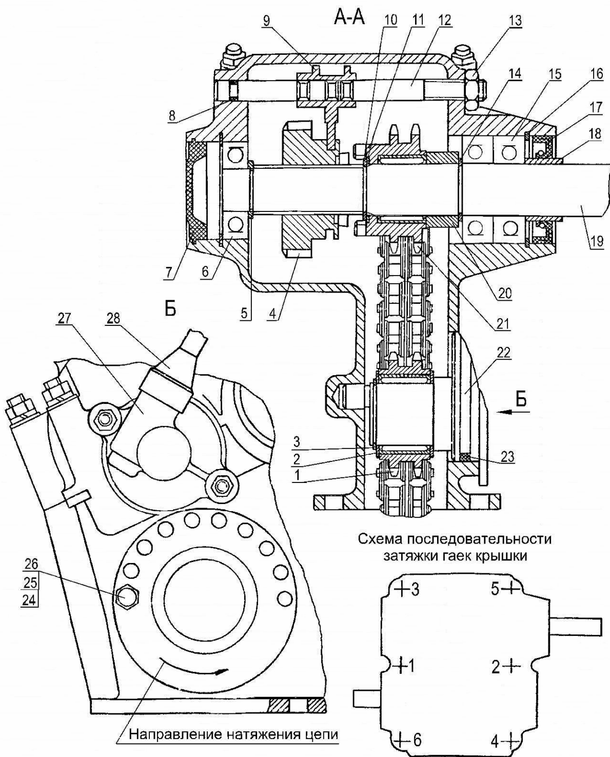
Рис. 5 – Коробка реверса
