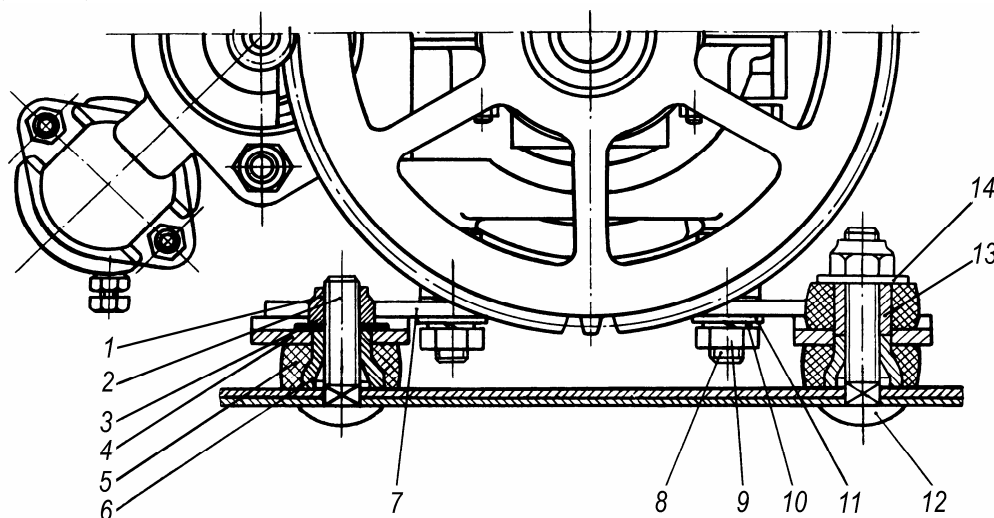
Рис. 3 – Подвеска двигателя
