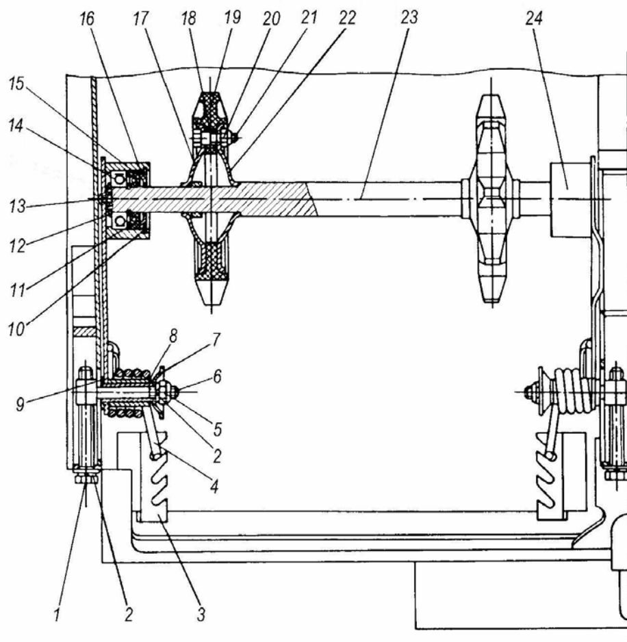
Рис. 7 – Направляющий вал с механизмом натяжения гусениц
