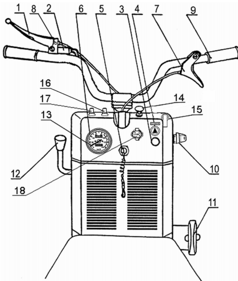
Рис. 9а – Органы управления (снегоход БУРАН АТЕ, АДТЕ)
