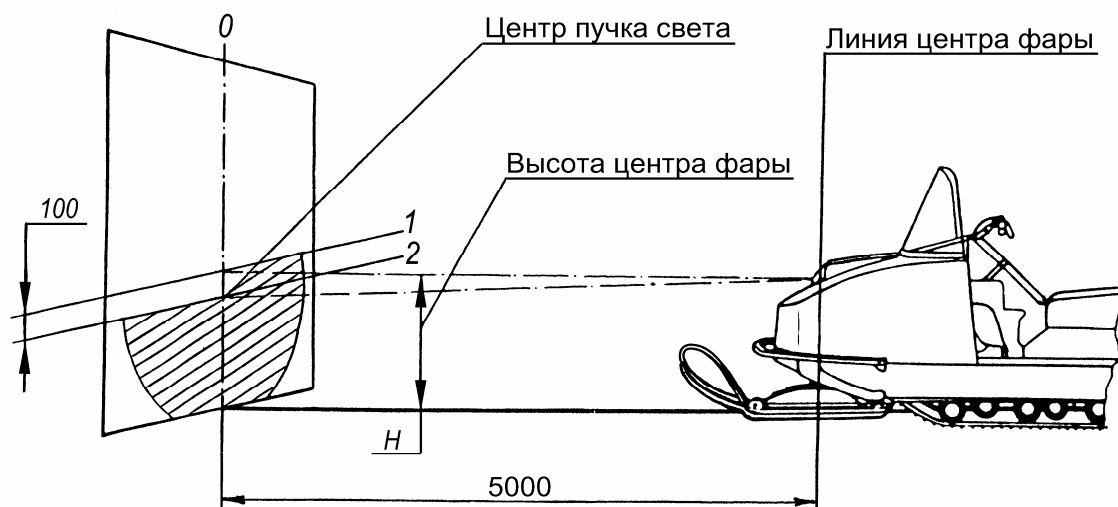
Рис. 23 – Регулировка фары
