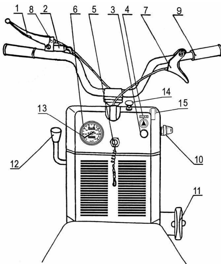
Рис. 9 – Органы управления (снегоход БУРАН А, АЕ, АД, АДЕ)
