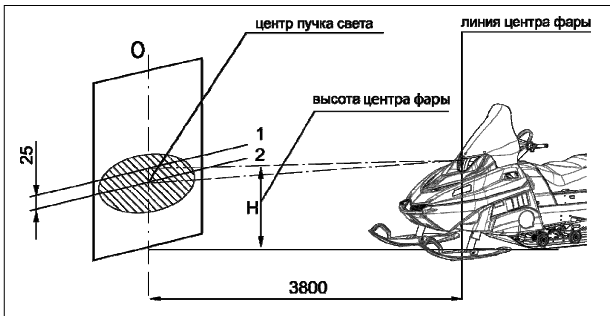
Рисунок 30 – Регулировка фары
