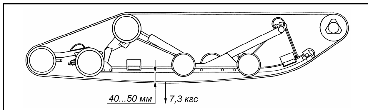
Рисунок 21 – Проверка натяжения гусеницы
