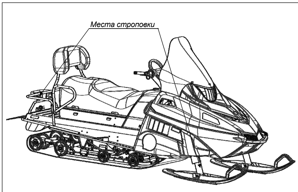
Рисунок 14 – Строповка снегохода
