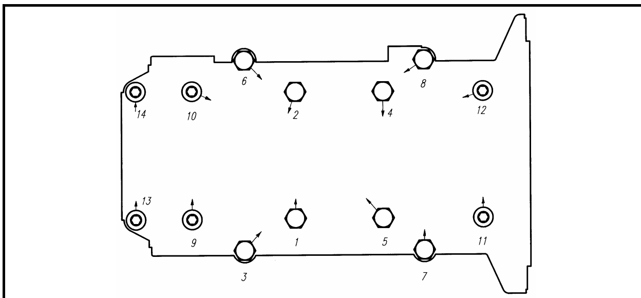
Рисунок 15 – Последовательность затяжки болтов и винтов крепления половин картера (двигатель с воздушным охлаждением)
