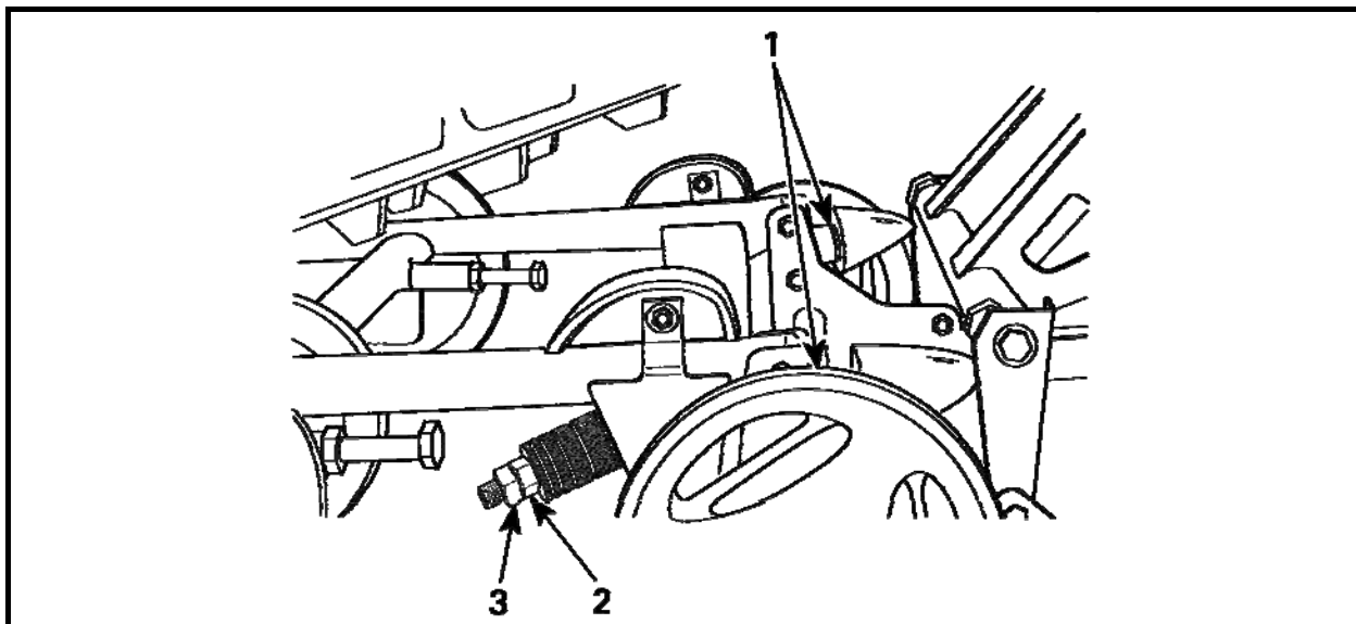
Рисунок 26 – Регулировка хода подвески
