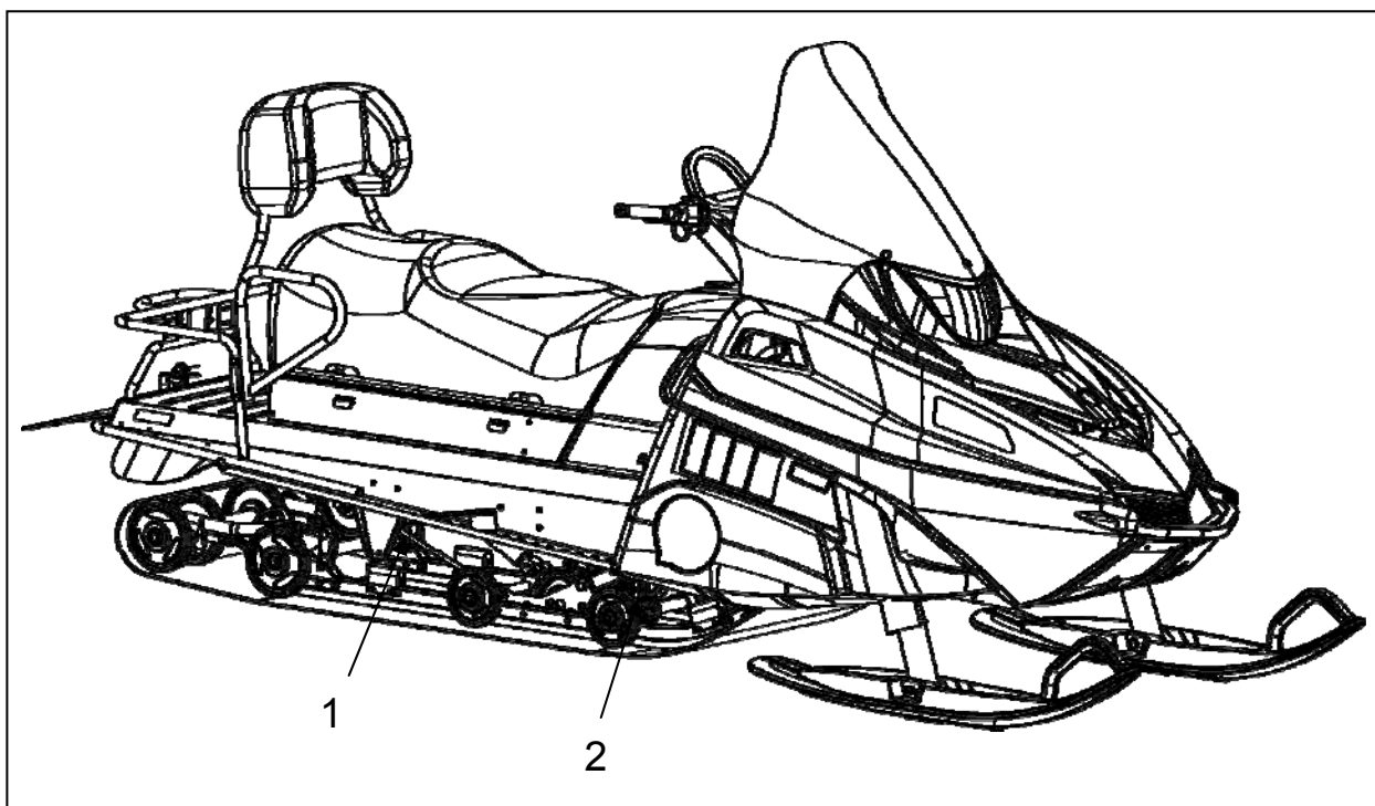
Рисунок 25 – Регулировка задней подвески
