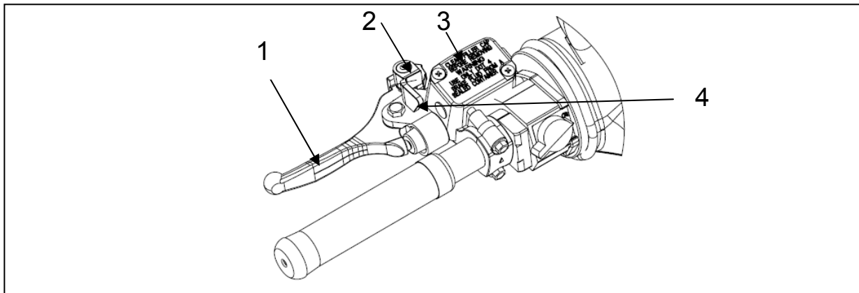
Рисунок 5– Расположение гидравлической тормозной системы и фиксатора стояночного тормоза
