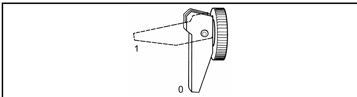
Рисунок 11 – Рычаг топливного корректора карбюратора
